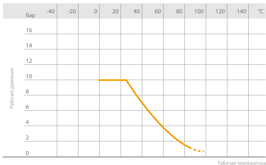
Рабочая температура
